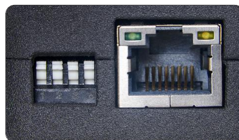
AE-1000設定スイッチ
